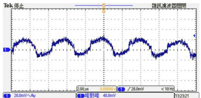
图 8: 出输出电压纹波与噪声(满载). (典型输入, 于输出端加 1μF MLCC 陶瓷电容)
