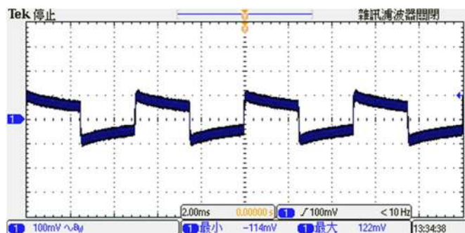
图 7: 进阶负载的输出变化 (典型输入, 于 50~70% 的 \Delta I_o/\Delta t = 1A/\mu s 输出电流)
