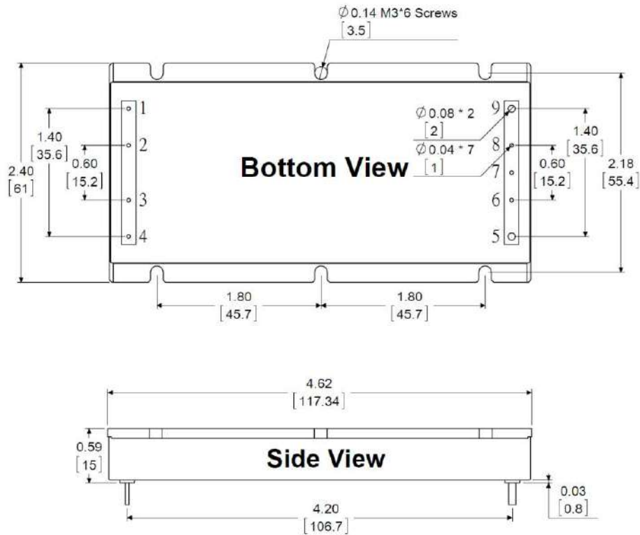
尺寸图-B (金属壳法兰片)
